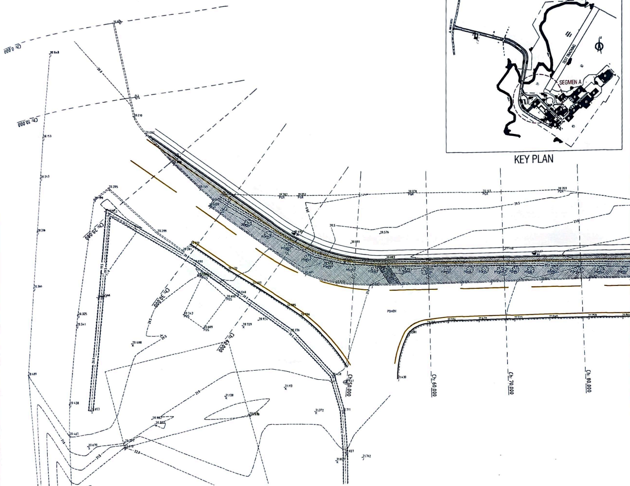
DETAIL PLAN LAYOUT SEGMENT A STA. 0+00 - STA. 0+80 SKALA 1 : 250
