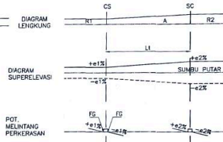
4 KURVA LINGKARAN - CLOITOID - LINGKARAN
