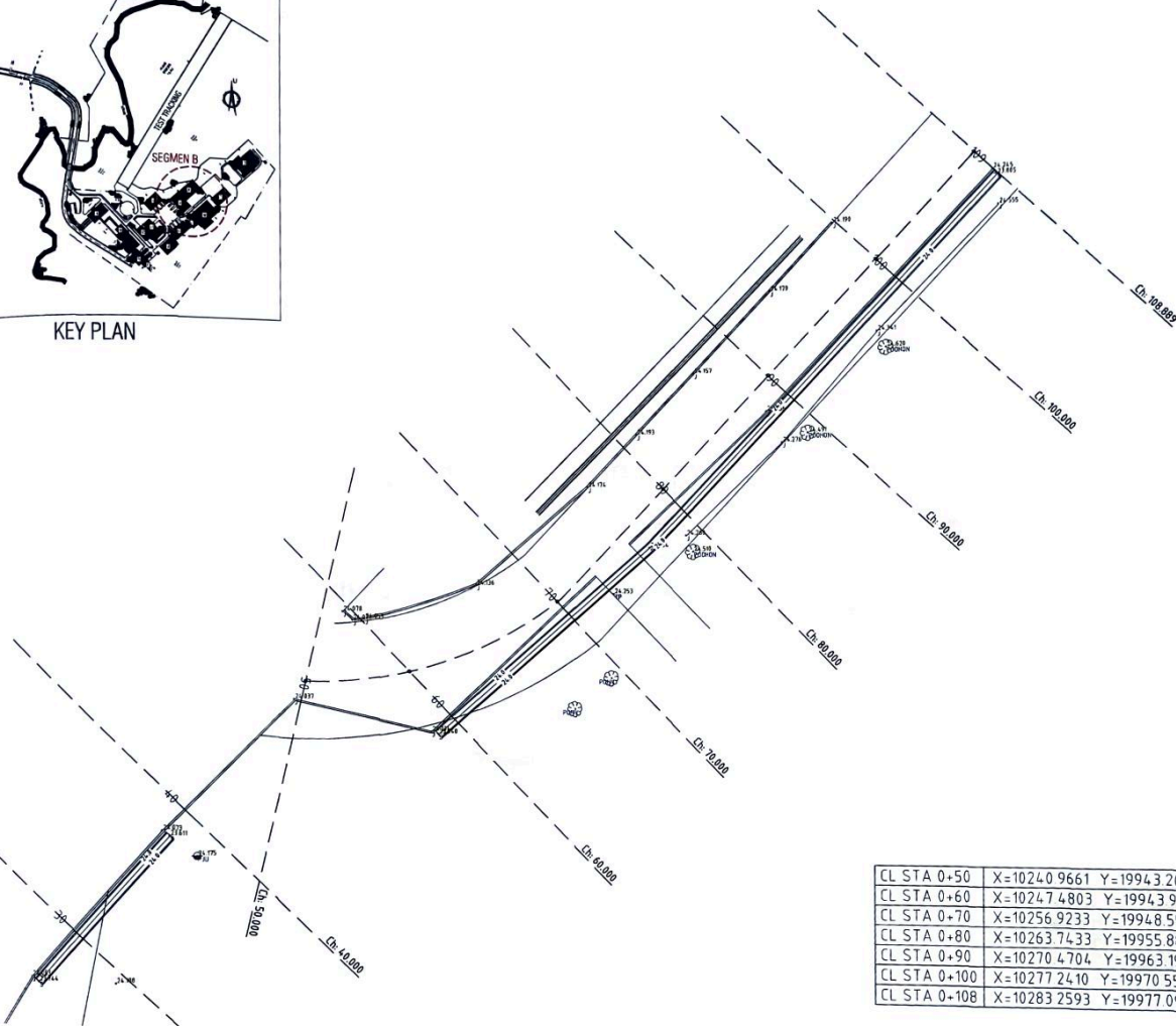
ALIGNMENT LAYOUT SEGMENT B STA. 0+80 - STA. 0+108
