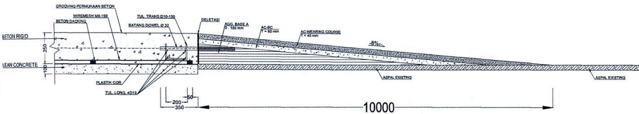
TYPICAL POTONGAN MEMANJANG JALAN SEGMENT E SKALA 1 : 200
