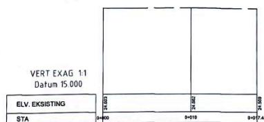
PLAN & PROFILE LAYOUT SEGMENT D STA. 0+00 - STA. 0+17 SKALA 1 : 150
