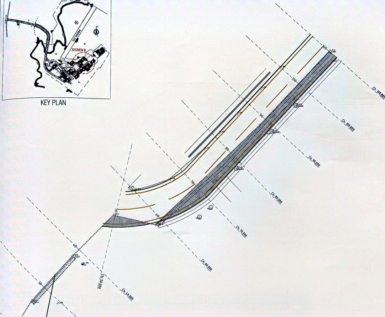
DETAIL PLAN LAYOUT SEGMENT B STA. 0+80 - STA. 0+108
