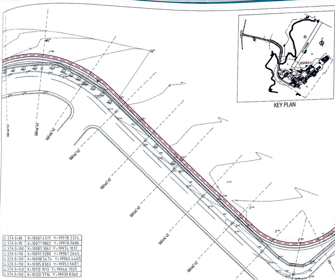
PLAN DRAINASE LAYOUT SEGMENT A STA. 0+80 - STA. 0+150
