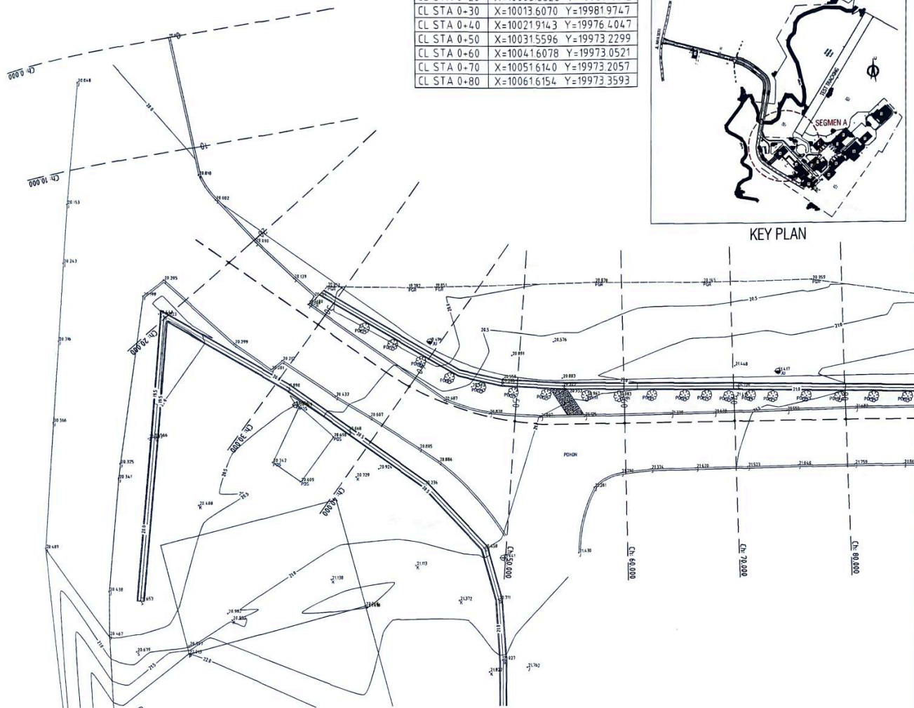
ALIGNMENT LAYOUT SEGMENT A STA. 0+00 - STA. 0+80
