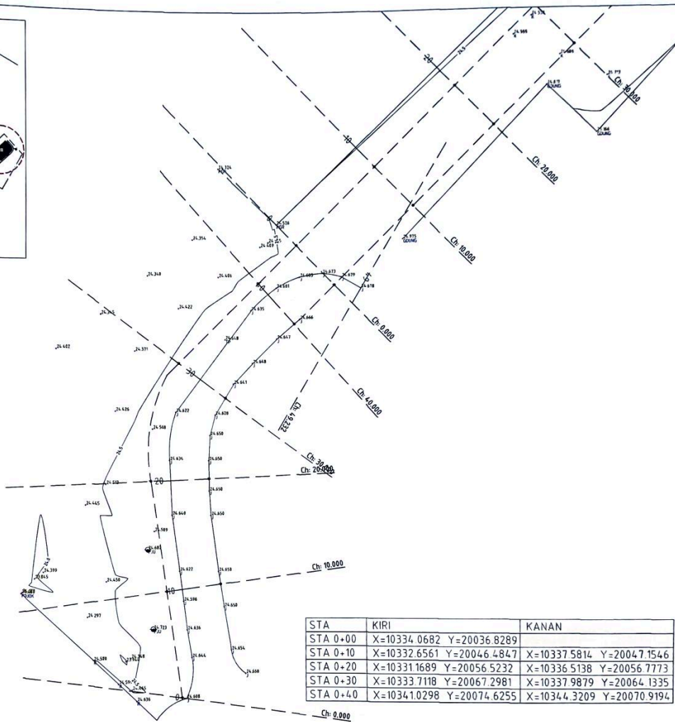
ALIGNMENT LAYOUT SEGMENT C STA. 0+00 - STA. 0+49
