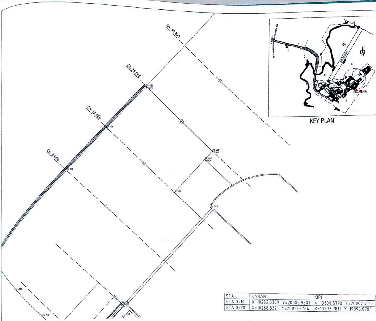
ALIGNMENT LAYOUT SEGMENT E STA. 0+00 - STA. 0+30
