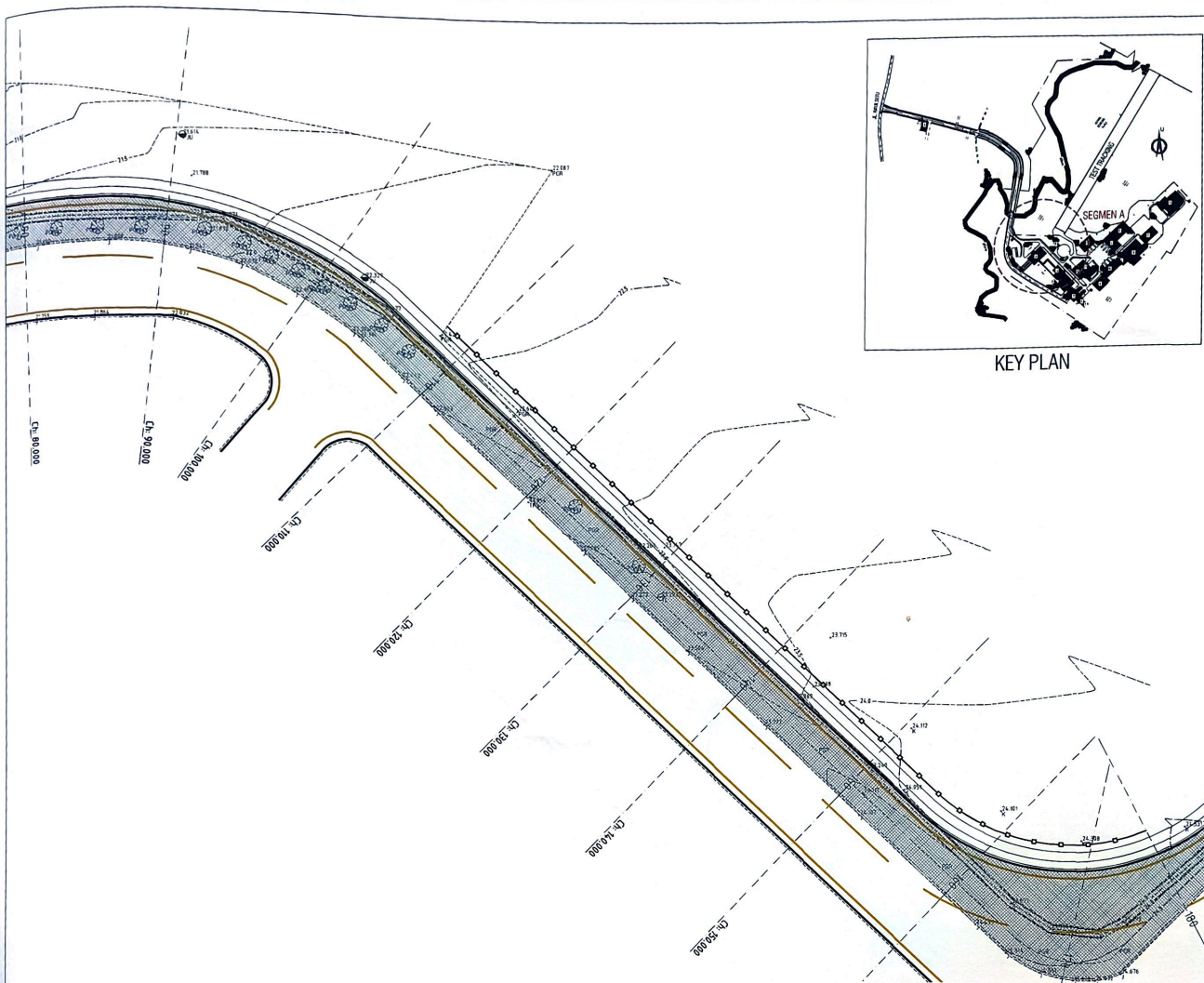
DETAIL PLAN LAYOUT SEGMENT A STA. 0+80 - STA. 0+150 SKALA 1 : 250
