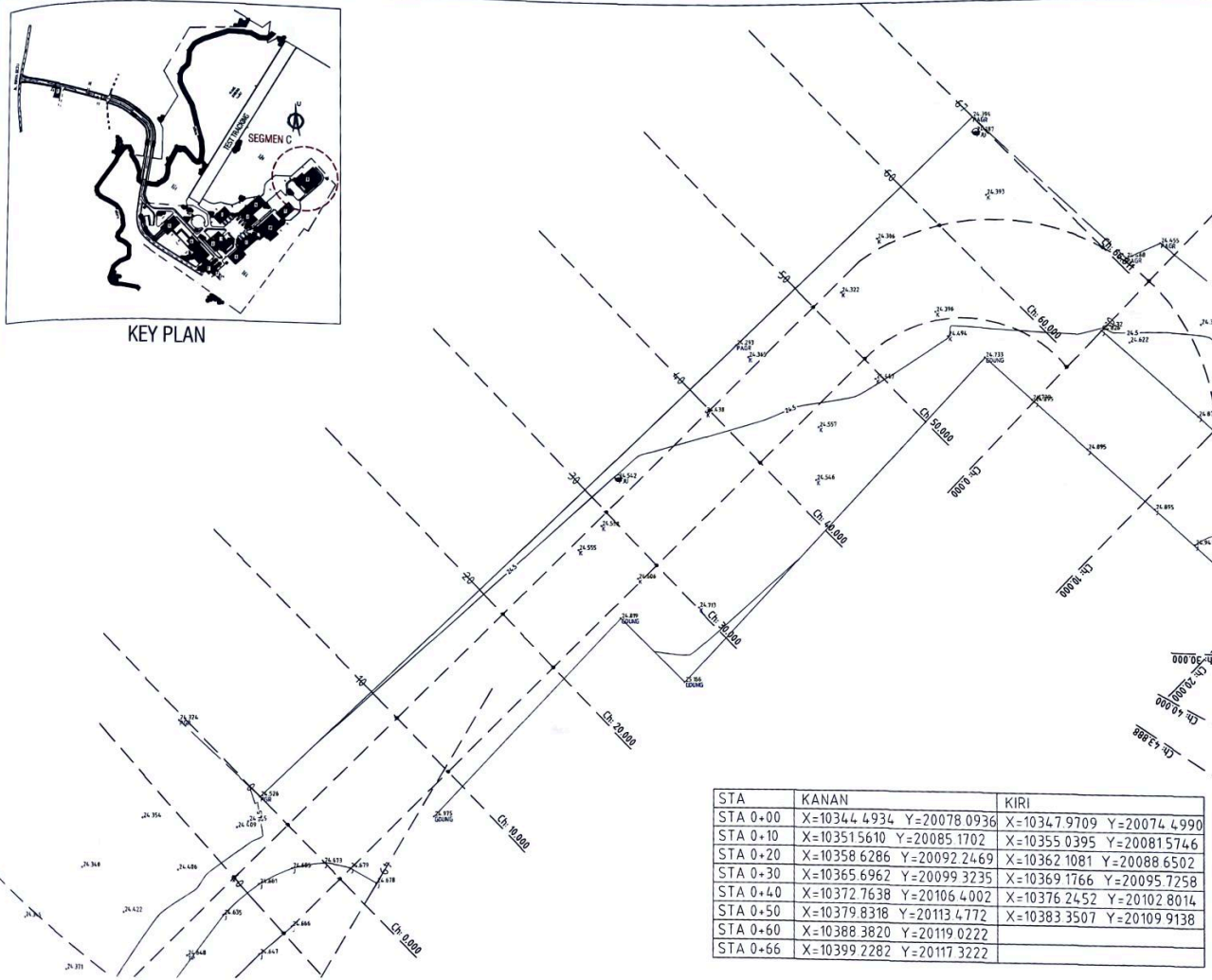
ALIGNMENT LAYOUT SEGMENT C STA. 0+00 - STA. 0+66
