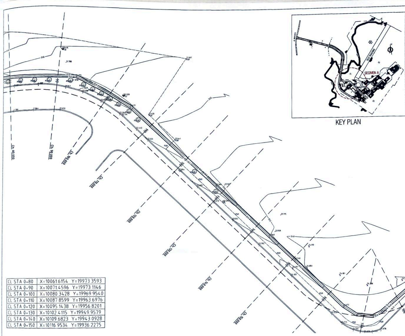
ALIGNMENT LAYOUT SEGMENT A STA. 0+80 - STA. 0+150 SKALA 1 : 250
