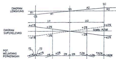
3 KURVA LINGKARAN - CLOITOID BOLAK BALIK - LINGKARAN
