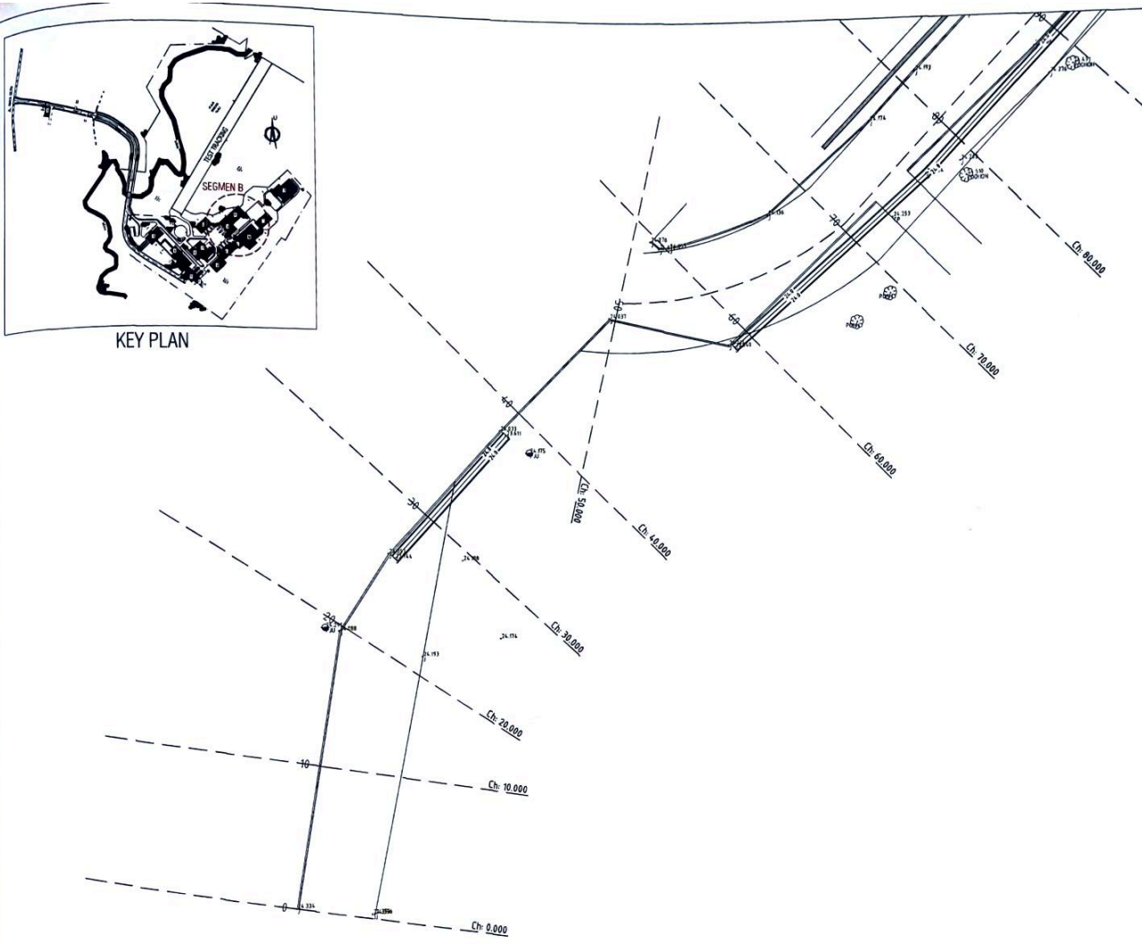
ALIGNMENT LAYOUT SEGMENT B STA. 0+00 - STA. 0+80 SKALA 1 : 250
