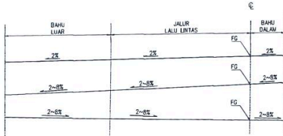
RAMP 1 LAJUR SATU ARAH
