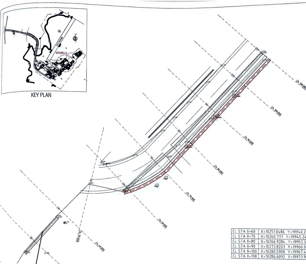
PLAN DRAINASE LAYOUT SEGMENT B STA. 0+80 - STA. 0+108
