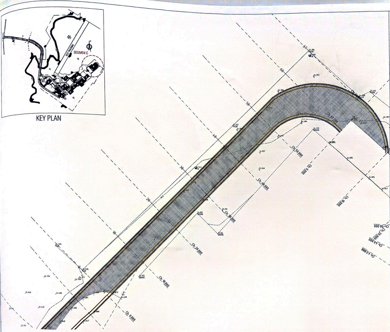
DETAIL PLAN LAYOUT SEGMENT C STA. 0+00 - STA. 0+66 SKALA 1 : 250
