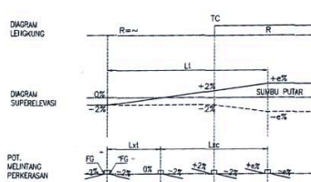
1 KURVA TANGEN - LINGKARAN TANPA LENGKUNG TRANSISI
