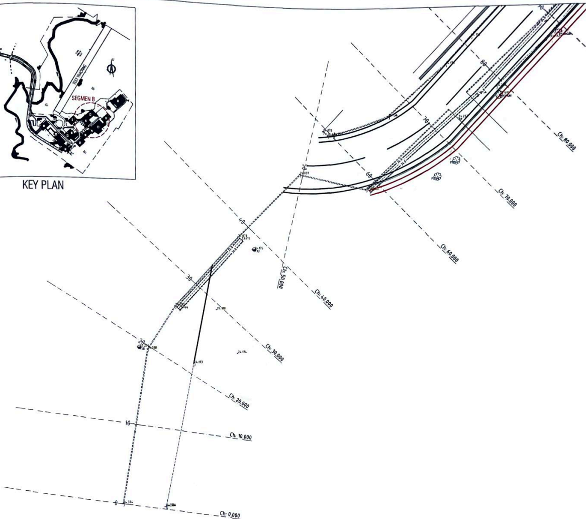
PLAN DRAINASE LAYOUT SEGMENT B STA. 0+00 - STA. 0+80
