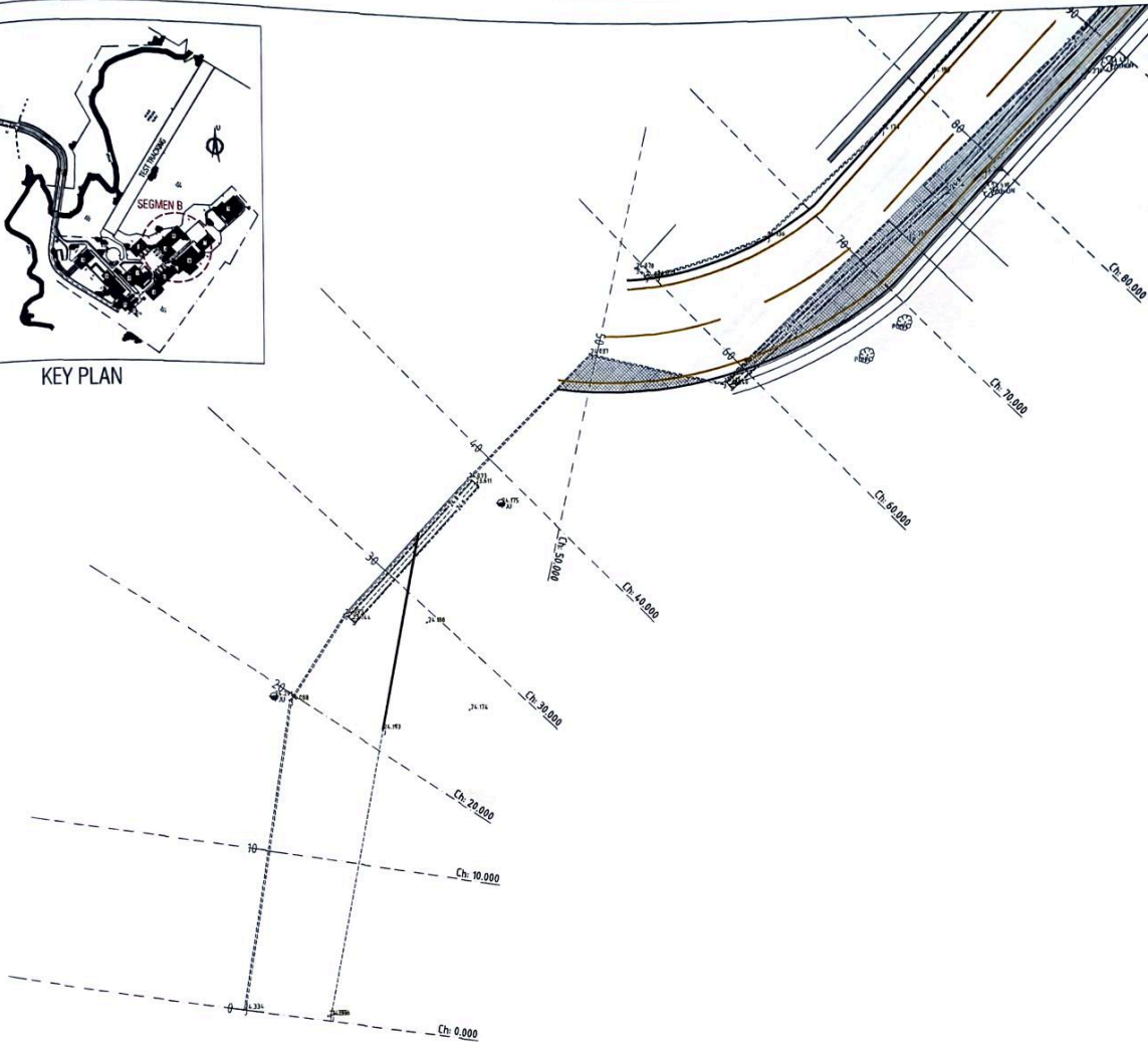
DETAIL PLAN LAYOUT SEGMENT B STA. 0+00 - STA. 0+80
