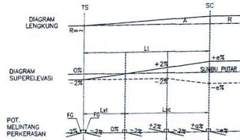
2 KURVA TANGEN - CLOITOID - LINGKARAN
